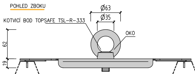
POHLED SHORA
