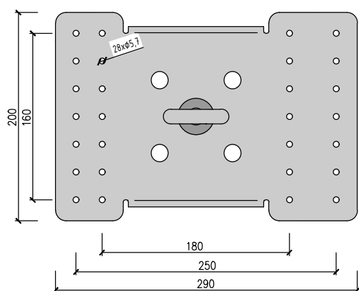
POHLED SHORA
